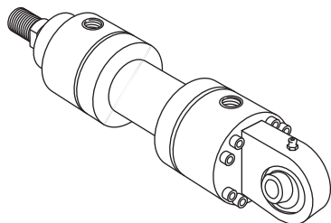
Befestigungsart MP5 Schwenkauge mit Gelenklager Boden
