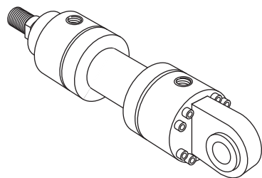
Befestigungsart MP3 Schwenkauge Boden
