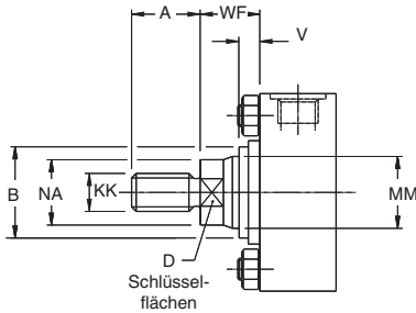
Stangenende, Ausführung 4
