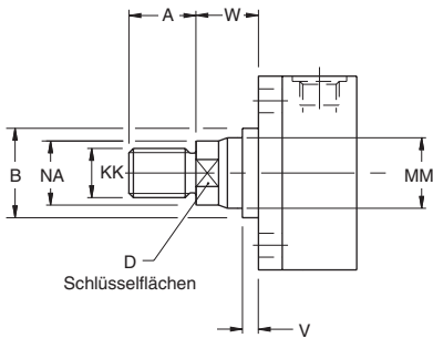
Stangenende, Ausführung 4
