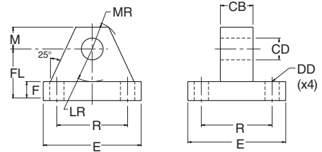
Montageplatte
