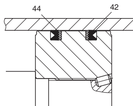
Lipseal-Kolben
