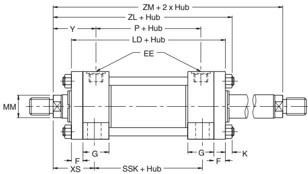
Zylinder mit beidseitiger Kolbenstange Bohrungsdurchmesser 38,1 mm bis 203,2 mm Lieferbar in den Typen TB, TD, J, JB, JJ, C, F, D, DD und G
