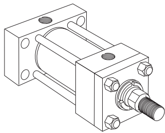
Typ HH Rechteckboden NFPA-Typ ME6
