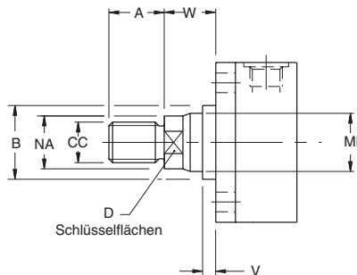
Stangenende, Ausführung 8
